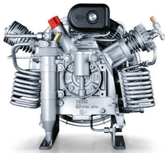
Bloc-compresseur IK 120 (utilisation dans PE-TE/TB, PE-HE, PE-MVE et PE-VE)
